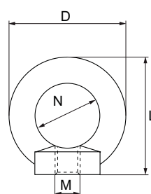
Ringmutter CM08EN
