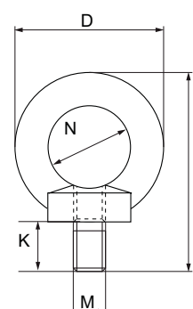
gyűrűcsavar CM08EB
